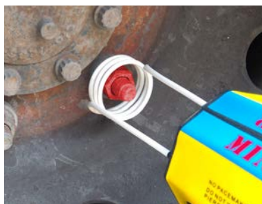
Smontaggio bulloni Disassembling bolts Desmontaje de pernos
